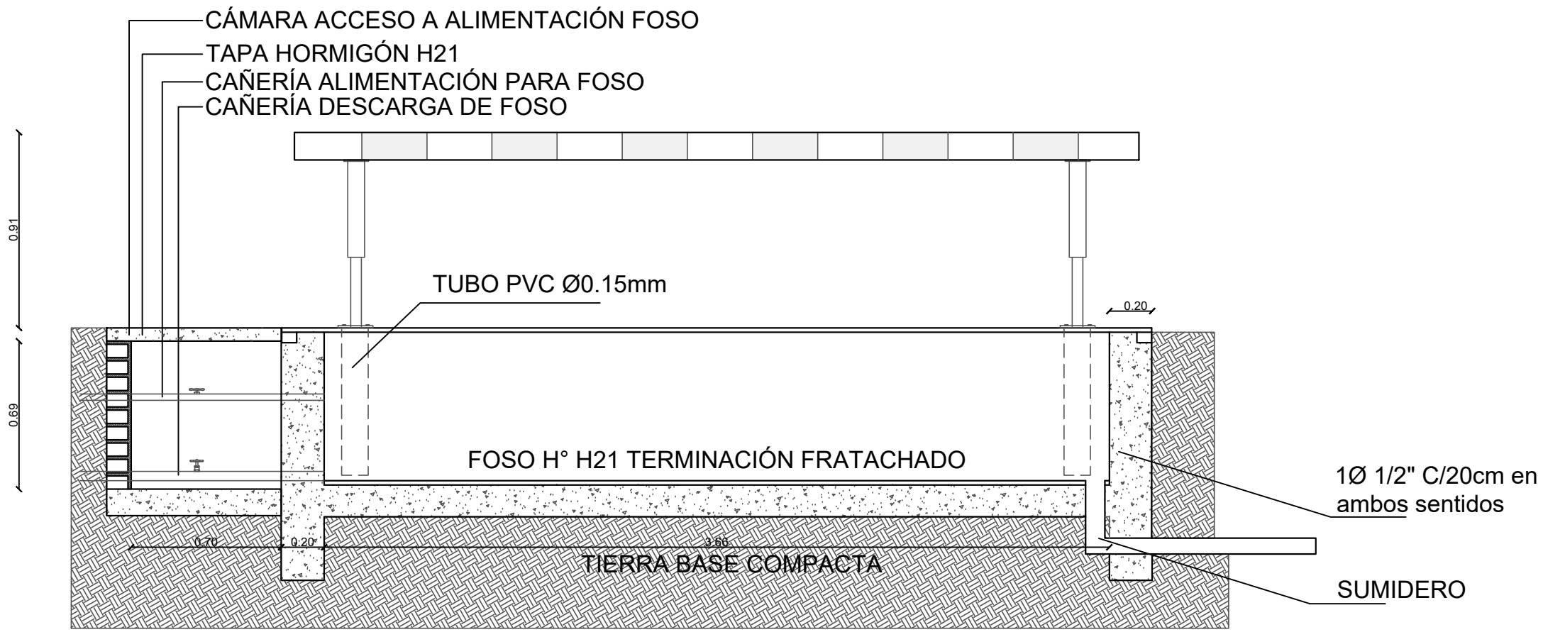
CORTE ESC 1:25
