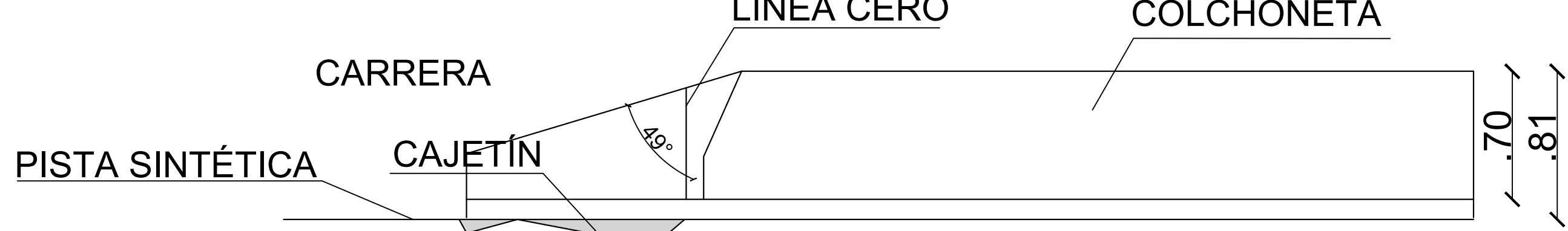
CORTE DETALLE CAJETÍN Y ZONA DE ATERRIZAJE ESC 1:25
