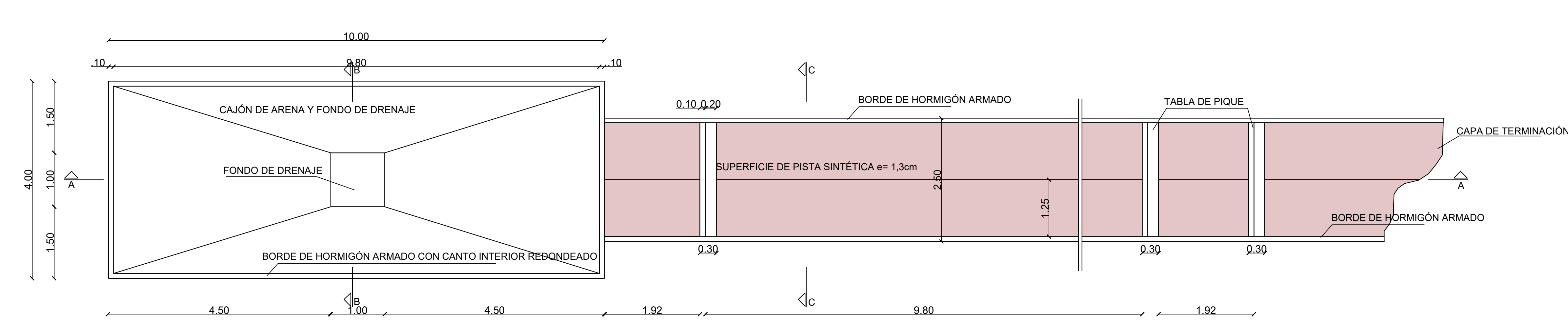
PLANTA ESC 1:50
