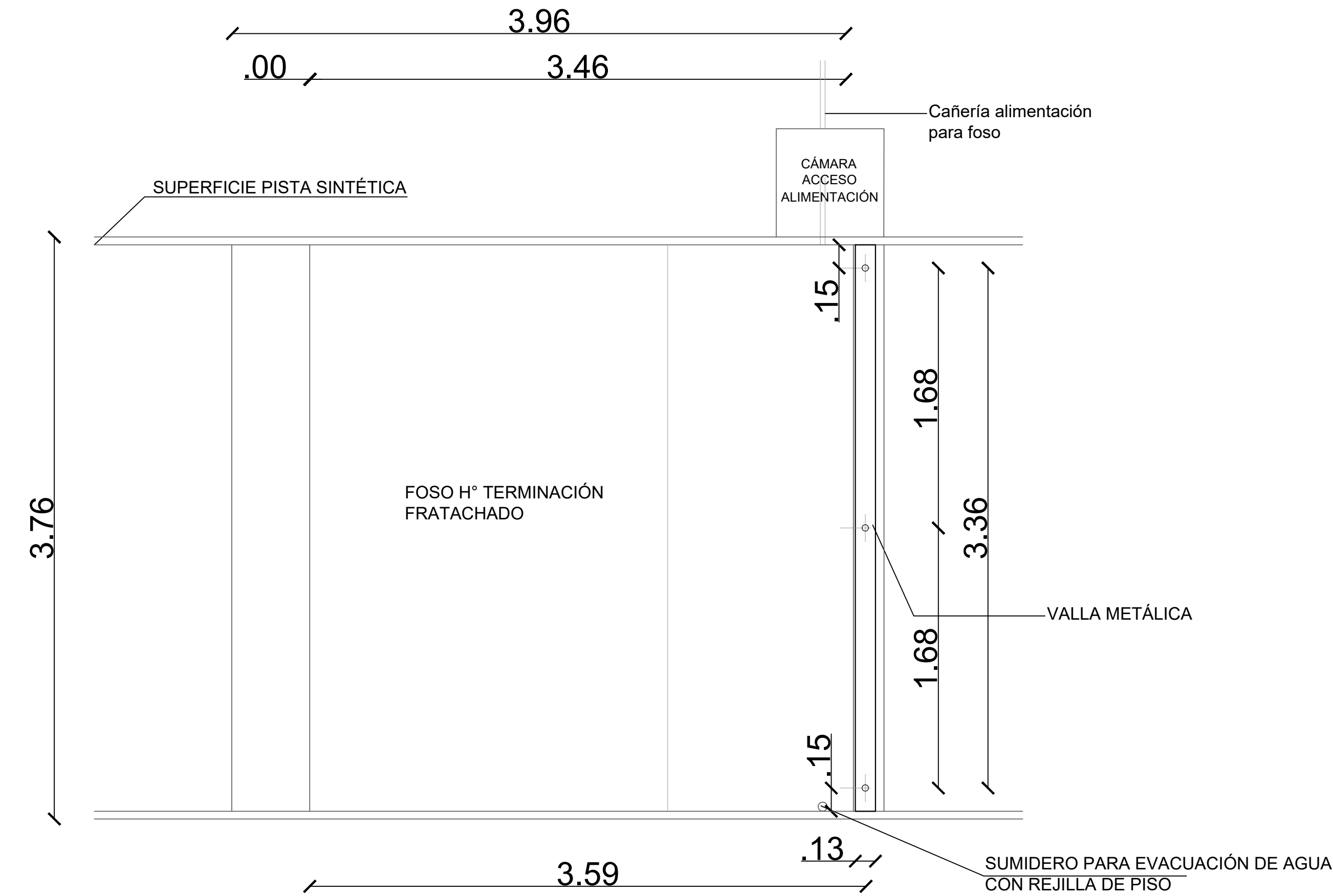
PLANTA ESC 1:25
