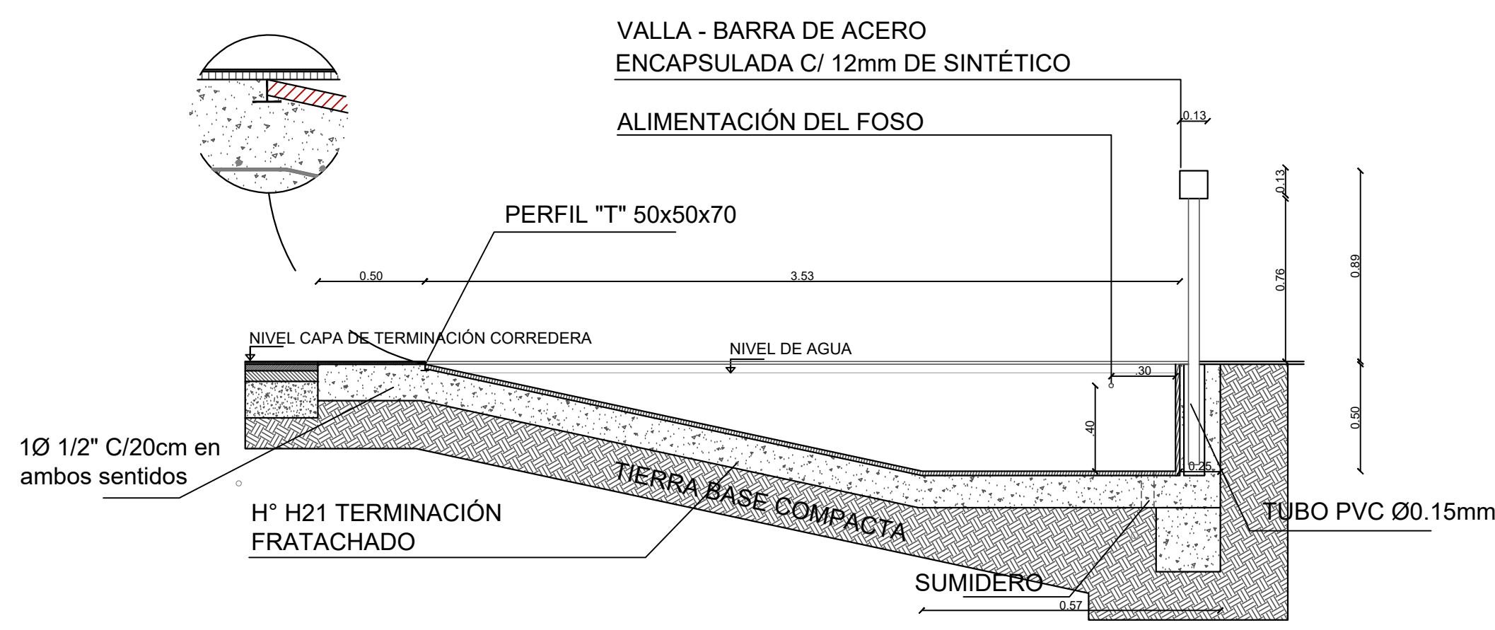
CORTE ESC 1:25
