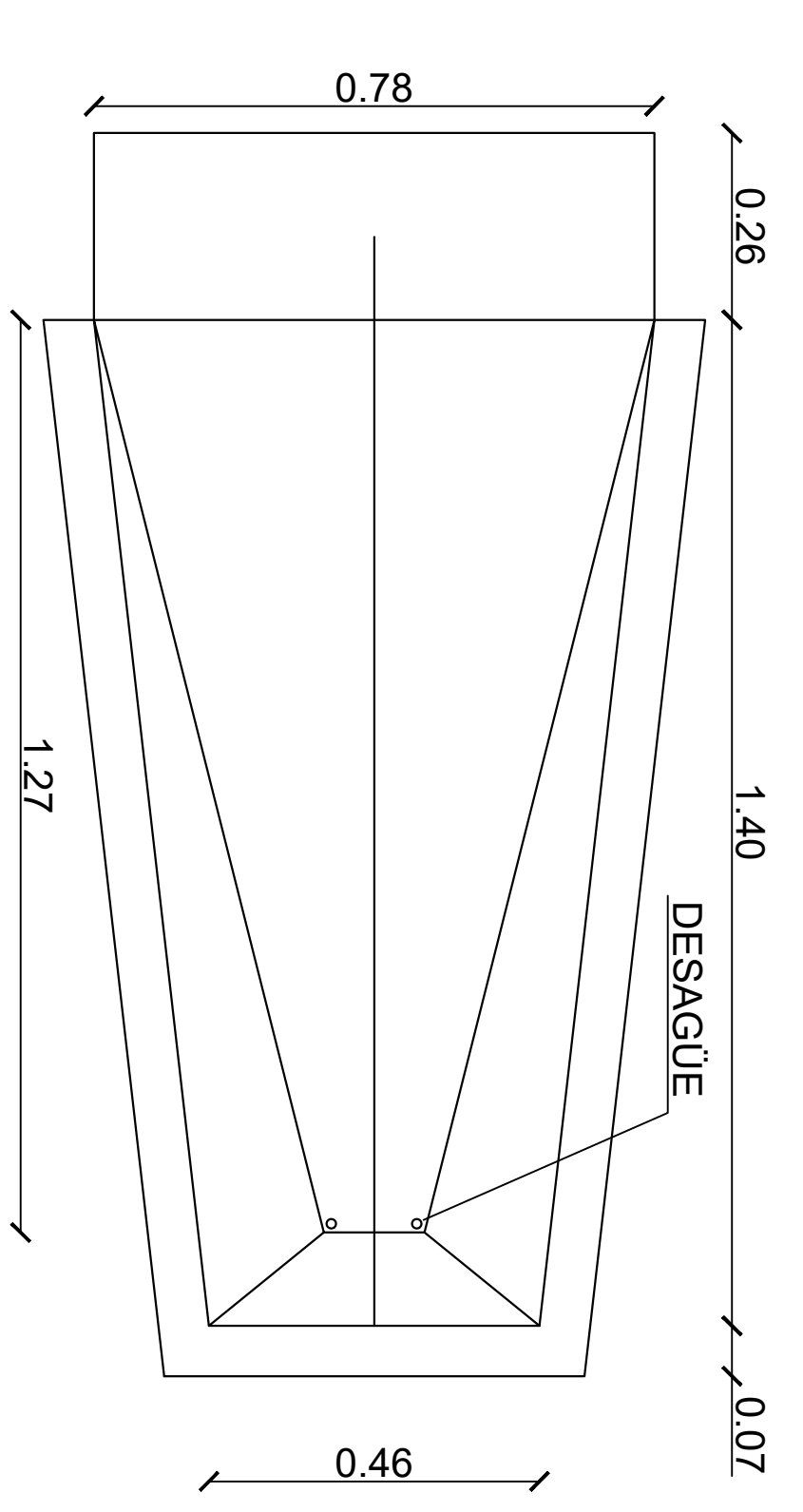
DETALLE CAJETÍN ESC 1:10
