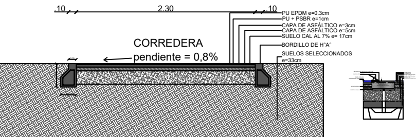
CORTE C-C ESC 1:50
