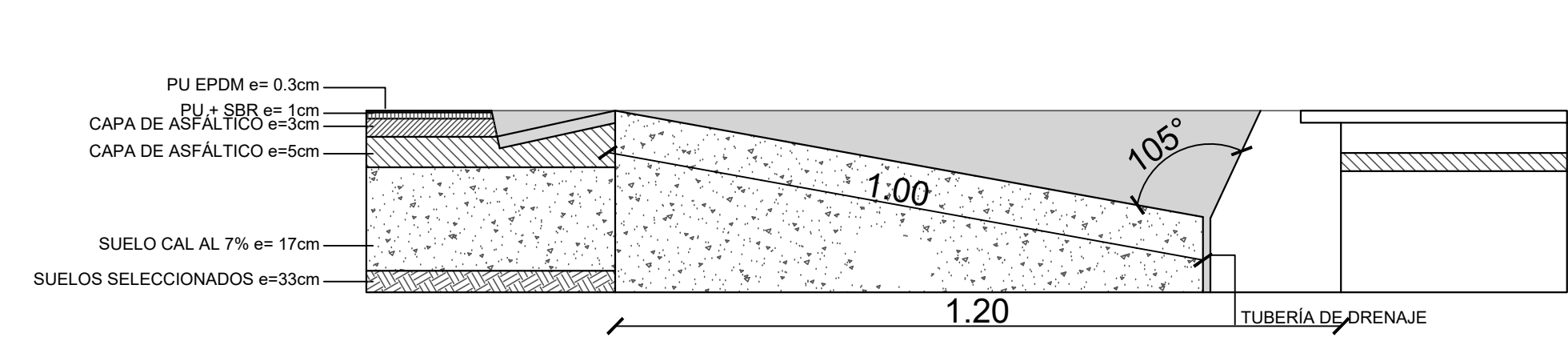
CORTE DETALLE CAJETÍN ESC 1:10
