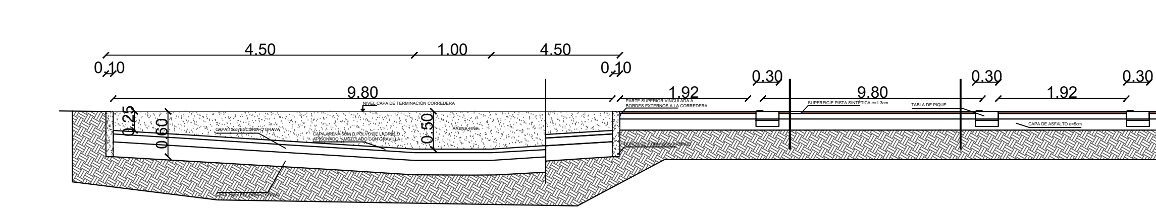
CORTE B-B ESC 1:50
