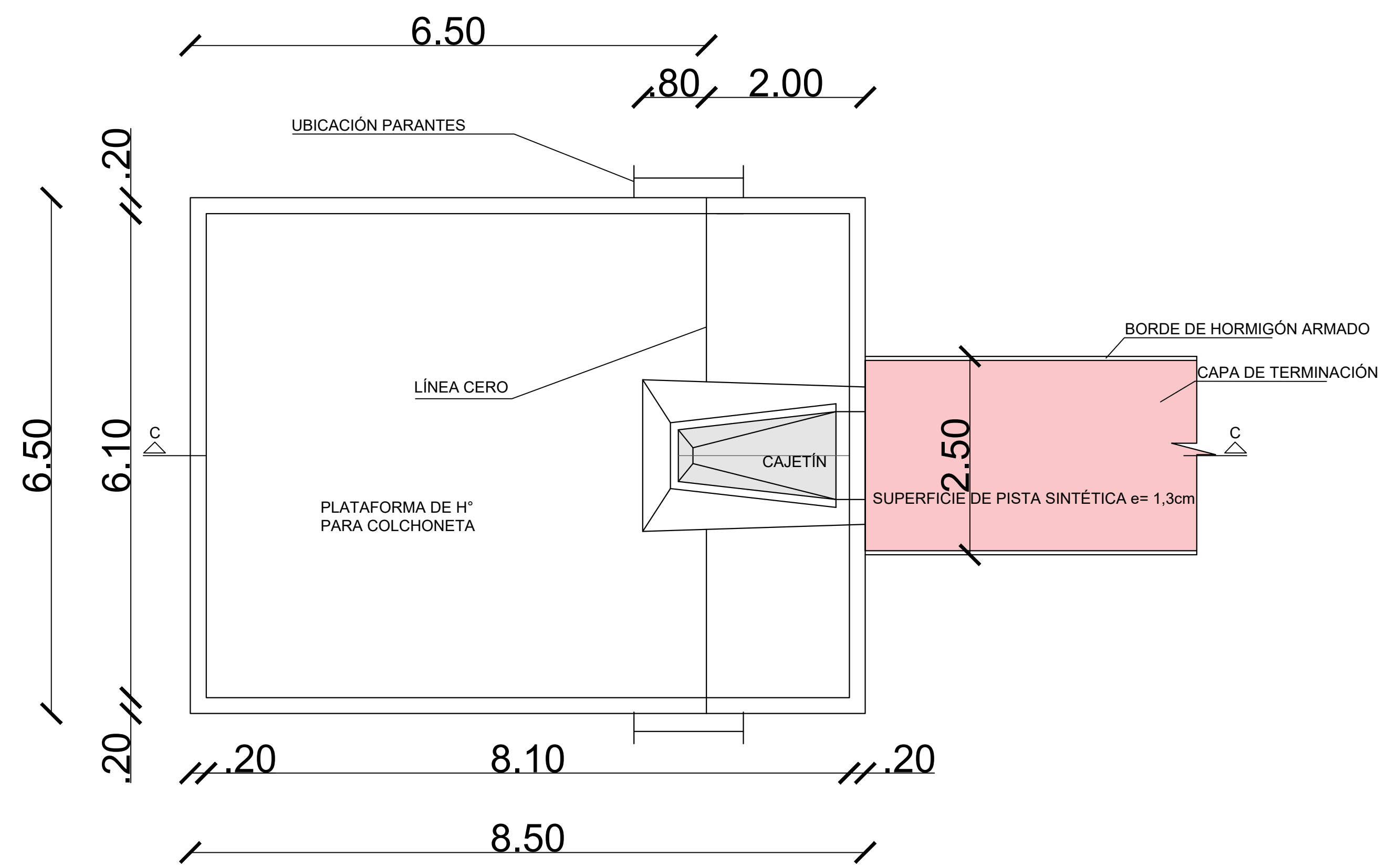
PLANTA ESC 1:50
