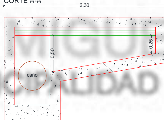
CORTE A-A
