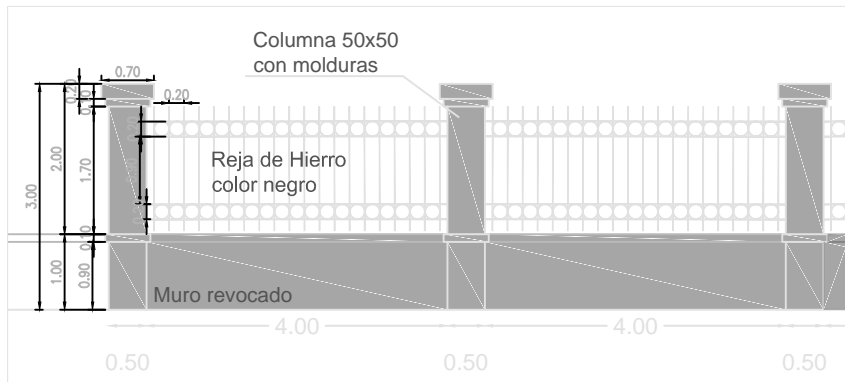
D01- DETALLE PARED REJA AV. BALBIN
