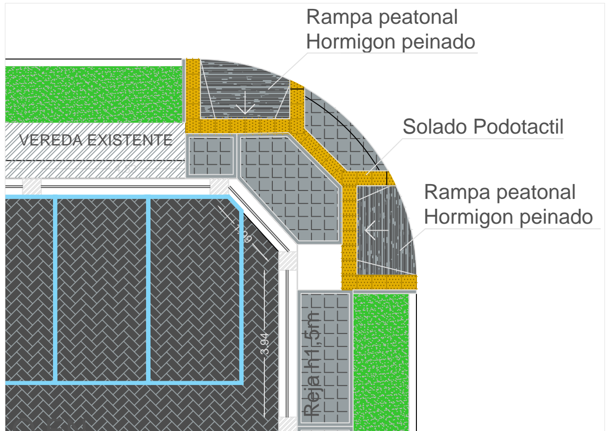
D02- DETALLE ESQUINA
